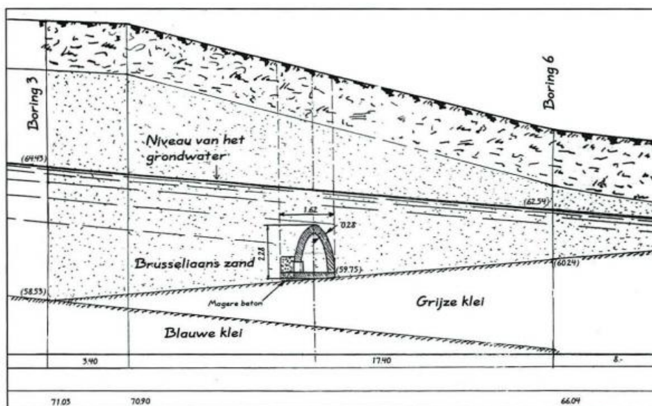
Doorsnede van het terrein waarin de galerij werd aangebracht.
