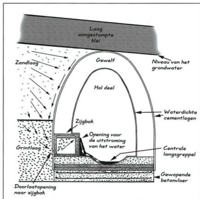
Doorsnede van de galerij voor wateropvang.
