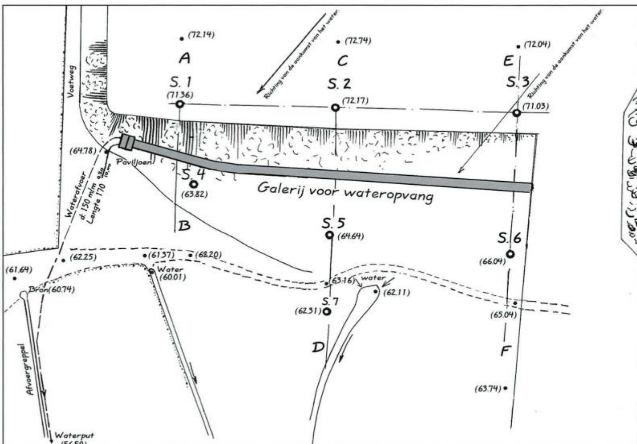
Plan van Jules Hennau met aanduiding (51-56) van de proefboringen en de bestaande bronnen. Aanduiding van de plaats van de aan te leggen galerij voor waterwinning.
